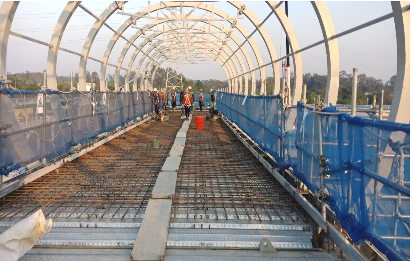
Thi công cầu đi bộ cho công nhân
